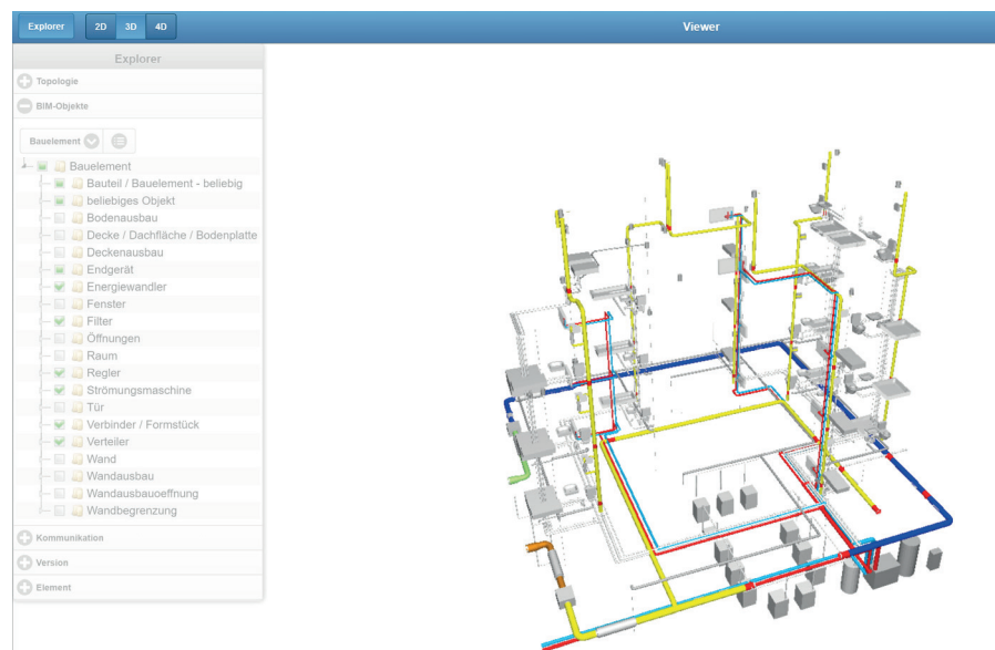
Fachplanung TGA in 3D im BIM4You-Viewer
